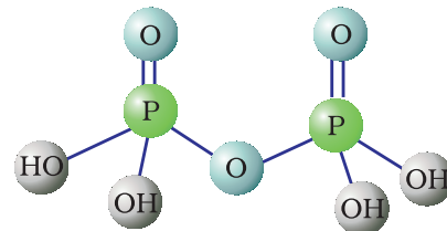
H_4P_2O_7 पायरोफॉस्फोरिक अम्ल
