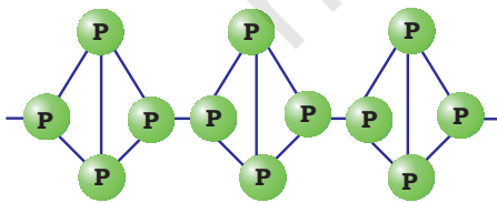
चित्र 7.3- लाल फॉस्फोरस
