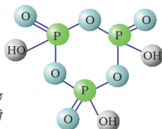
(HPO_3)_3 साइक्लोट्राइमेटाफॉस्फोरिक अम्ल
