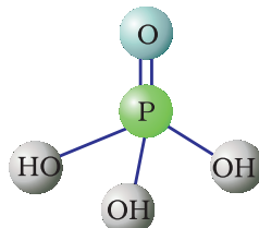
H_3PO_4 आर्थोफॉस्फोरिक अम्ल
