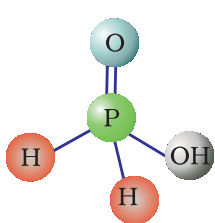
H_3PO_2 हाइपोफॉस्फोरस अम्ल
