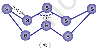
चित्र 7.5 (क) विषमलंबाक्ष सल्फर में S 8 वलय
