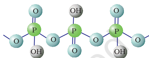
(HPO_3)_3 पॉलीमेटाफॉस्फोरिक अम्ल
